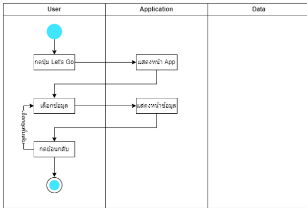
ภาพ 6 รูปการออกแบบการใช้งานหน้าข้อมูล
