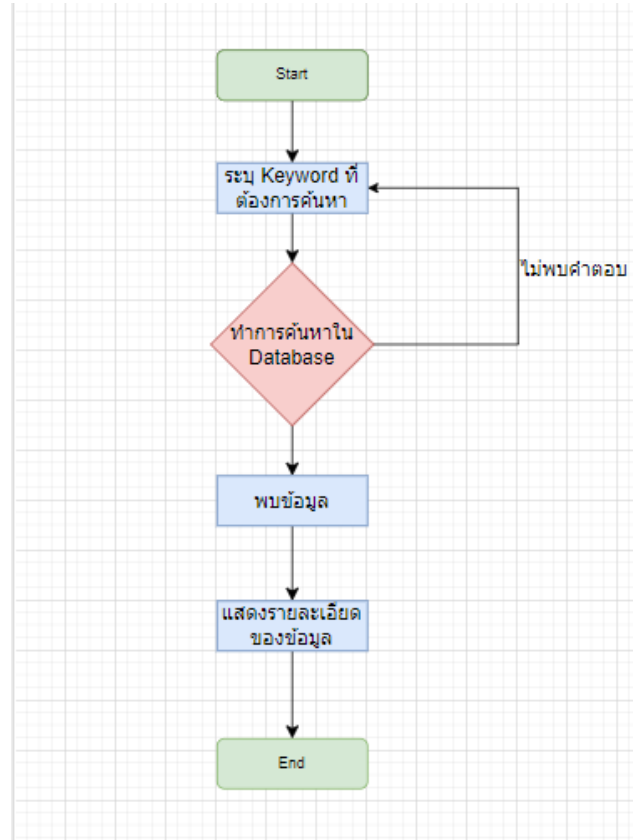
ภาพ 9 รูปวิธีการค้นหา
