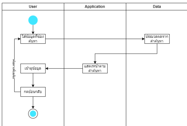
ภาพ 7 รูปการออกแบบการค้นหา
